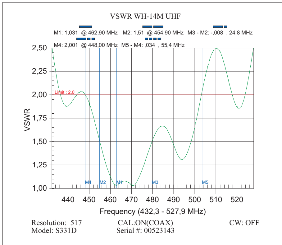
Типовое КСВ для F(C)=462,9 МГц
