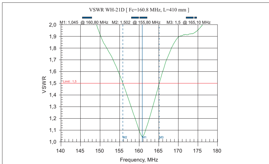
Типовое КСВ для F(C)=160,8 МГц
