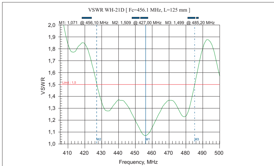
Типовое КСВ для F(C)=456,1 МГц
