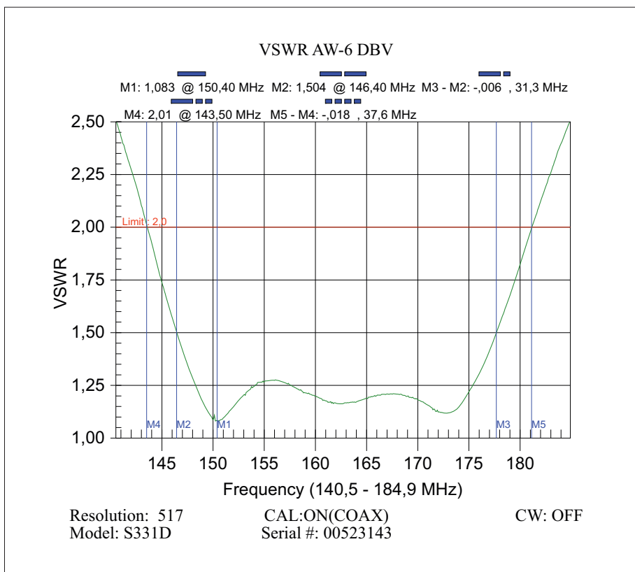
Типовое КСВ для F(C)=150,4 МГц на креплении MC-1UHF
